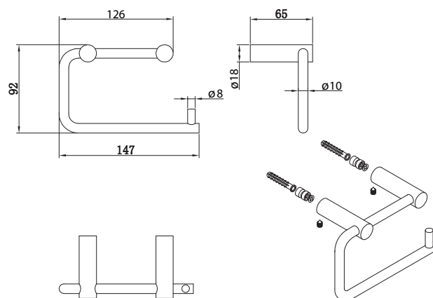
Schéma technique
