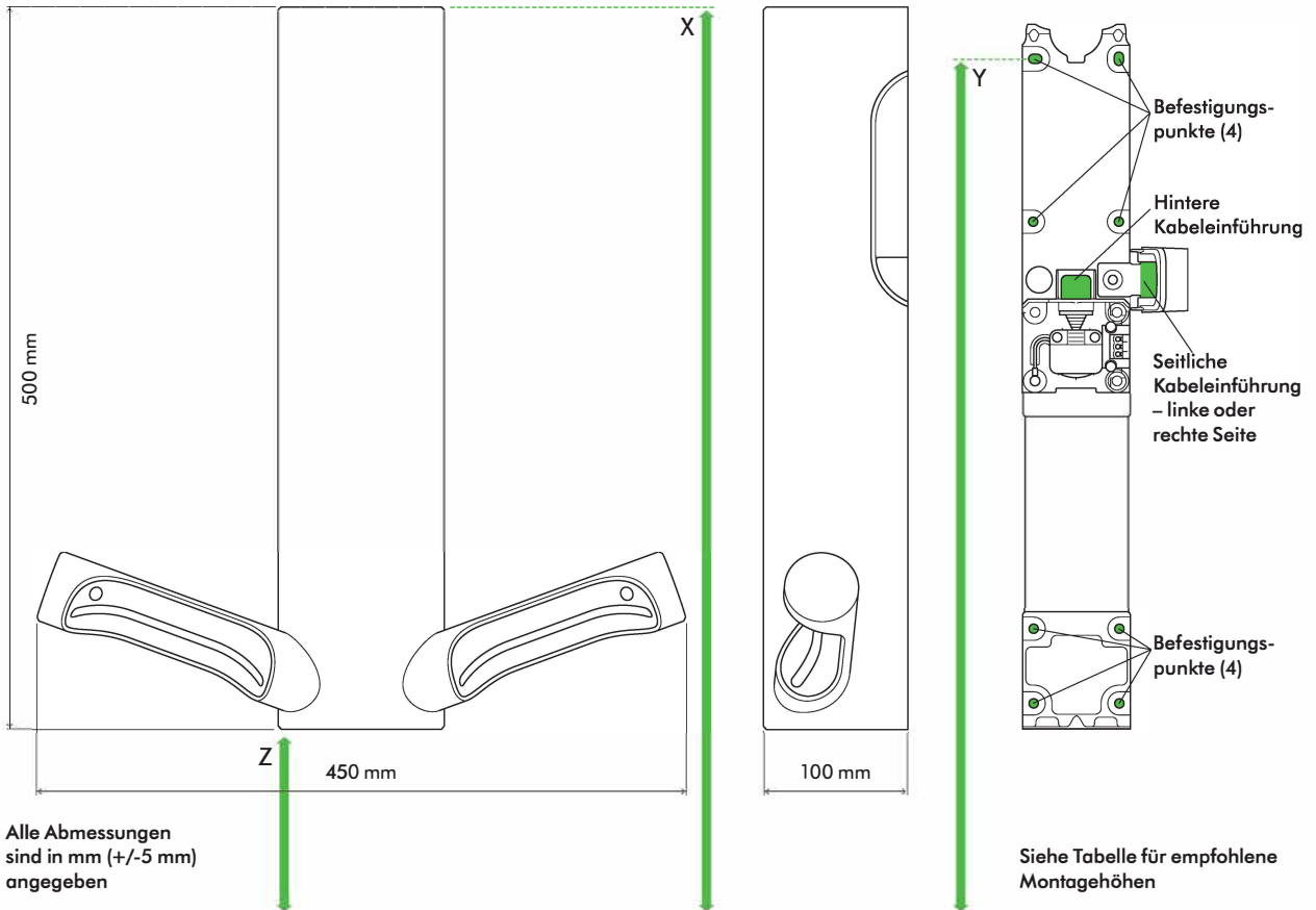
Vorderansicht
